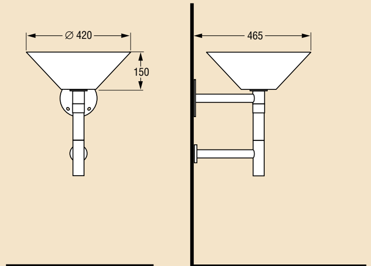
PO4K,18 Pollux Waschtisch Pollux washbasin
